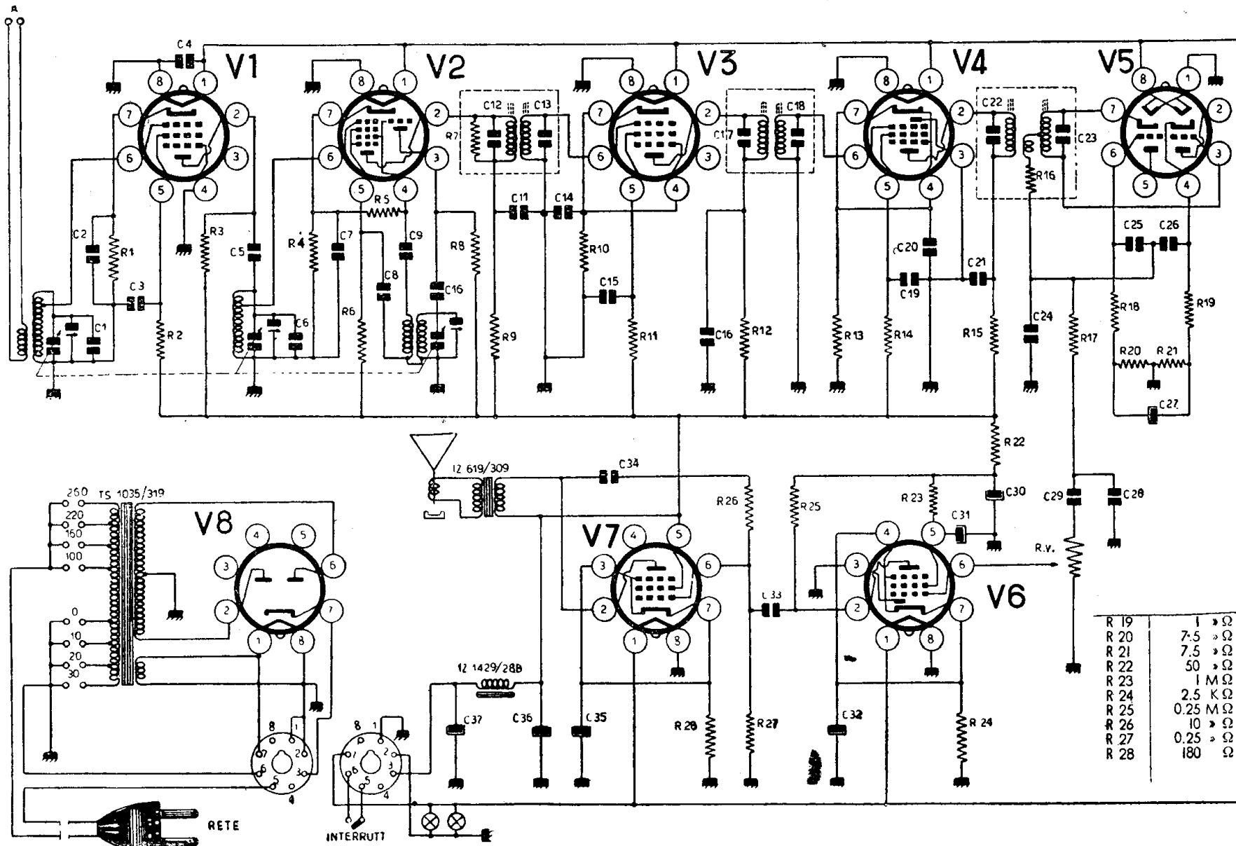
PHONOLA RADIO - Mod. MF 801 - Ricevitore a sola modulazione di frequenza. Gamma 88-108 Mc. Media frequenza 10,7 Mc. V1 amplif. RF, V2 miscelatrice, V3 e V4 amplif. MF, V5 rivelatrice a rapporto, V6 e V7 amplif. BF. Potenza 4 W.
